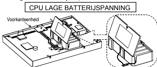
Figuur 10. Batterijvervanging
