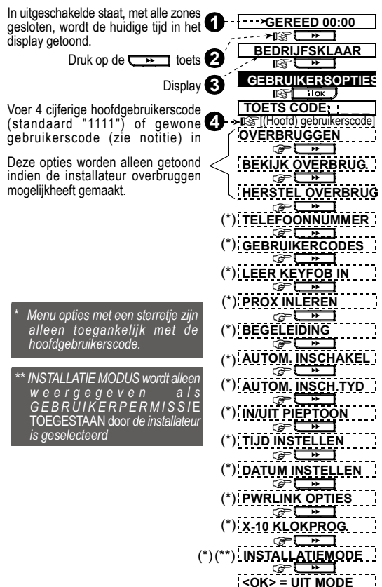
Figuur 7 - Het gebruikerinstellingen menu openen
