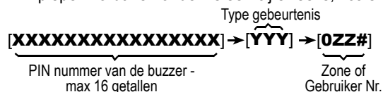
Figuur 6. Pieperbericht structuur
