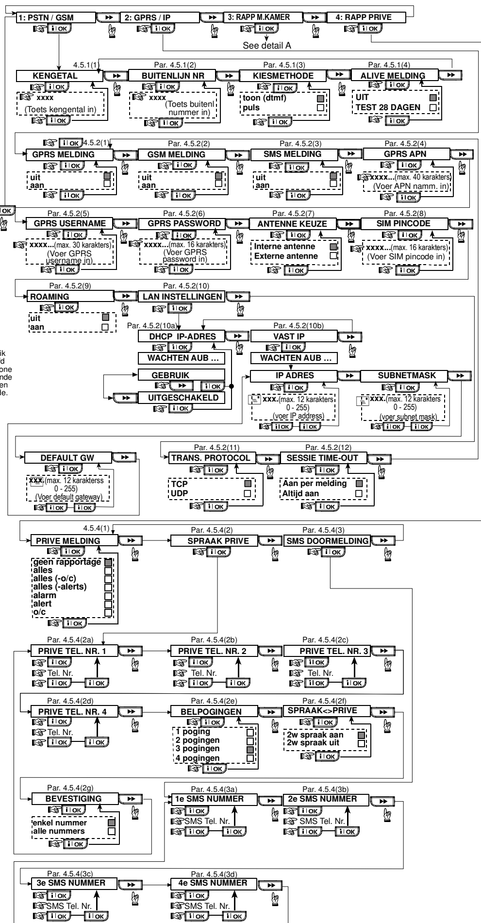
Figuur 4.5 – COMMUNICATIE PARAMETERS definiëren
