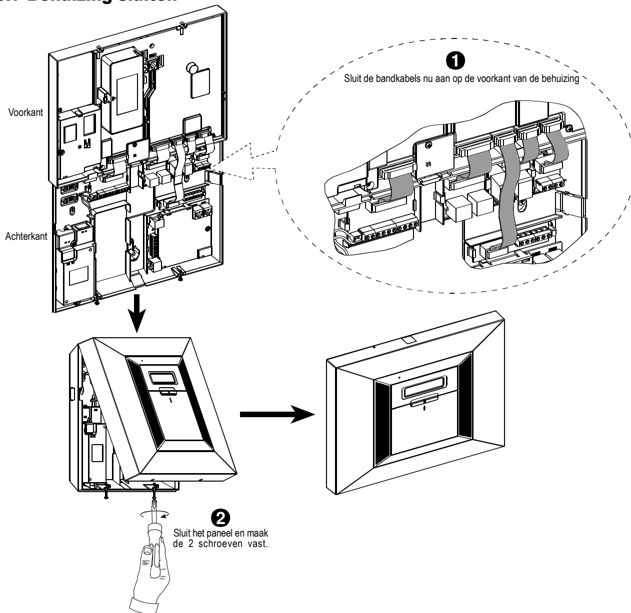
Figuur 3.1k – Behuizing sluiten
