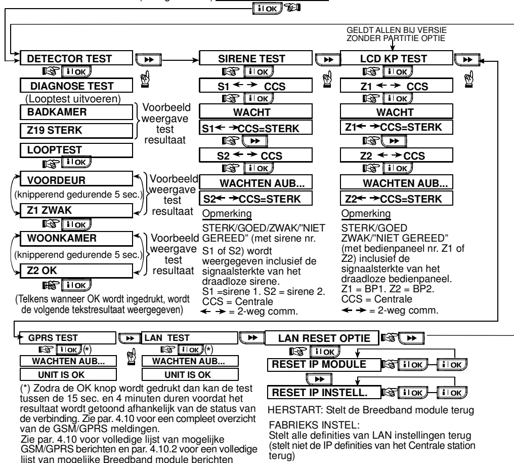
Figuur 4.10 – Test schema
