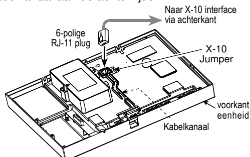
Figuur 3.1i - X-10 Interface module aansluiting
