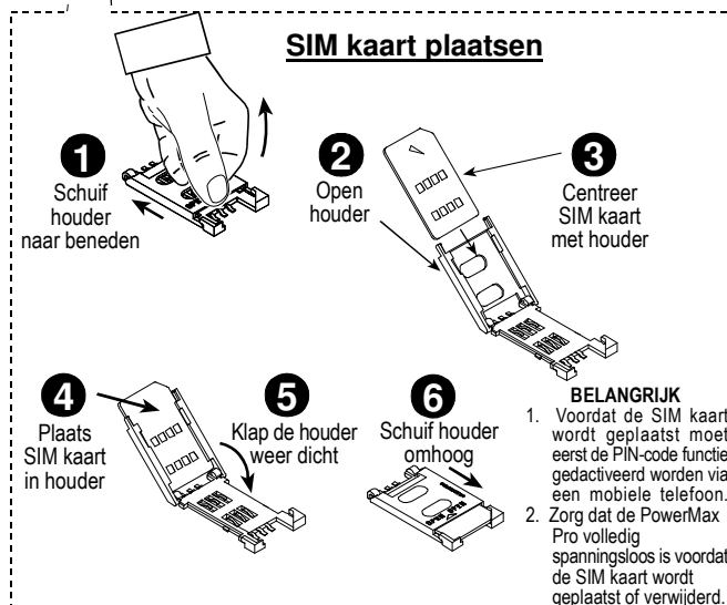
Figuur 3.1j - Optionele GSM/GPRS module montage
