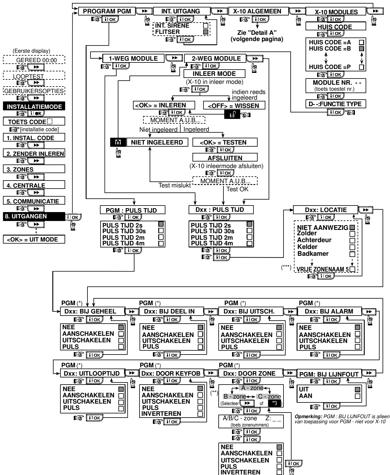
Figuur 4.8 – Schema uitgangen definiëren
