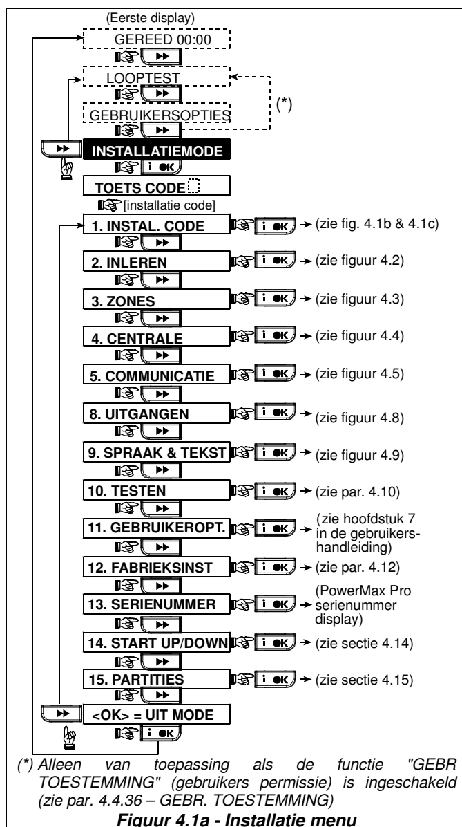
Figuur 4.1a - Installatie menu
