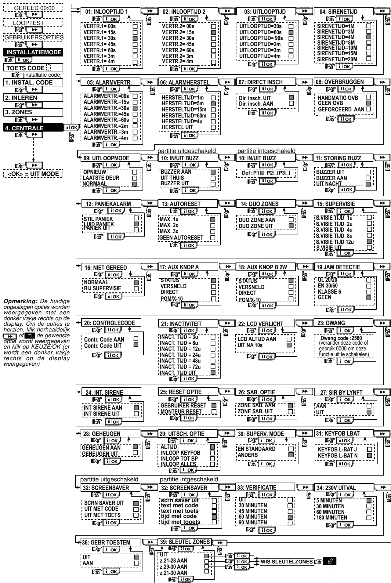
Figuur 4.4 – SYSTEM PARAMETERS programmeerschema
