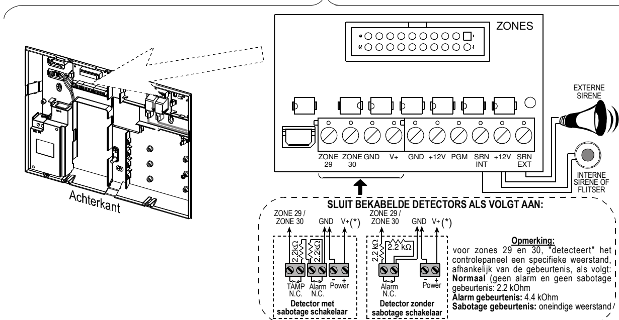
Figuur 3.1c – Zone en Sirene bedrading
