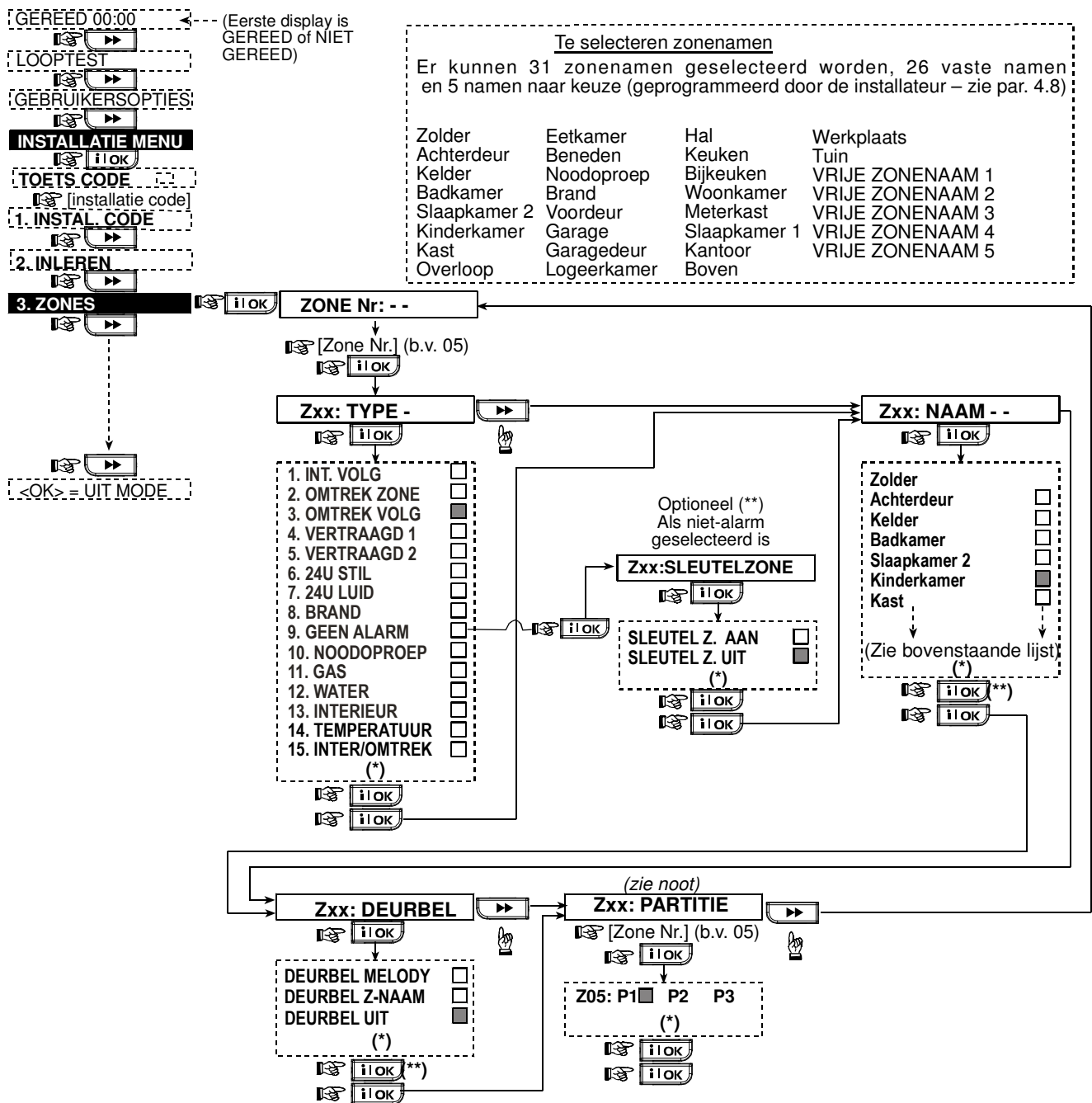
Figuur 4.3 - Zone programmeerschema
