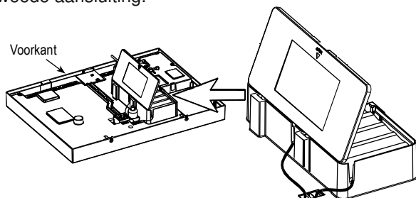
Figuur 3.1h – Batterypack plaatsen
