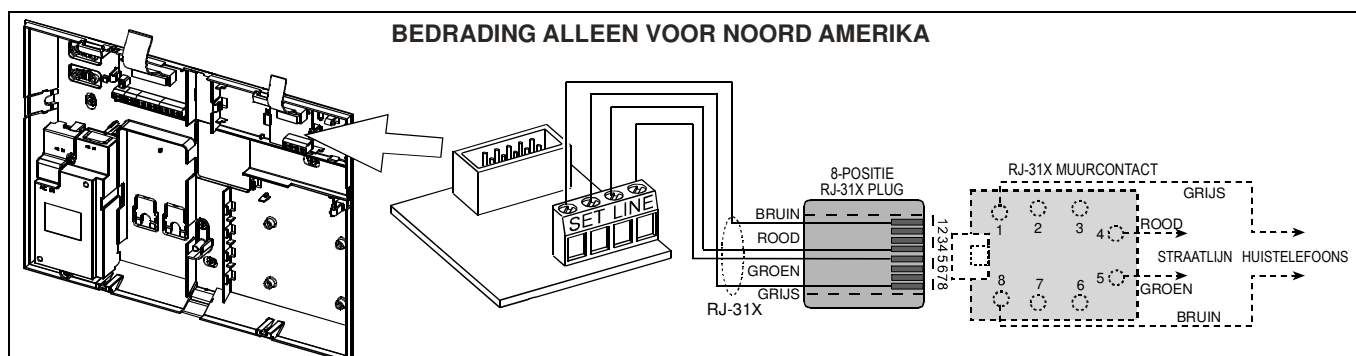
Figuur 3.1b – Telefoon bedrading
