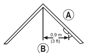
Figuur 7. Aanbevolen Plaats voor rookmelders in kamers met schuine plafonds.
