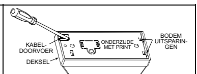
Figuur 5. De bovenkant losmaken
