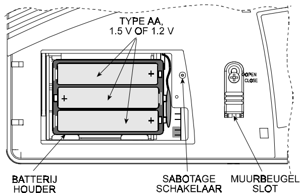
Figuur 13. Batterij compartiment en batterij houder
