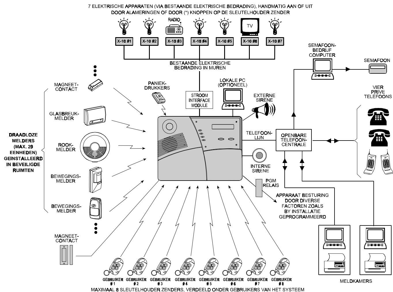
Fig. 2. Een typische configuratie
