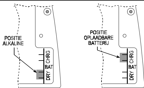
Figuur 13. Batterij jumper posities
