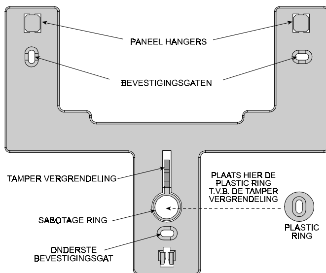
Figuur 8. Muurbeugel, voor aanzicht
