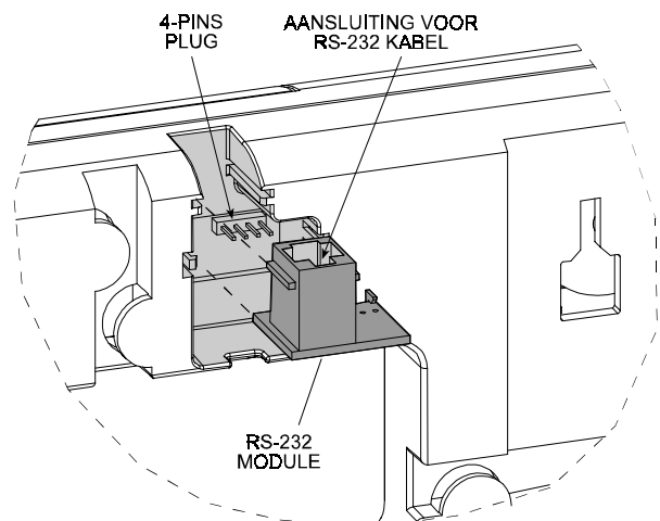
Figuur 28. Inserting de RS232 Module
