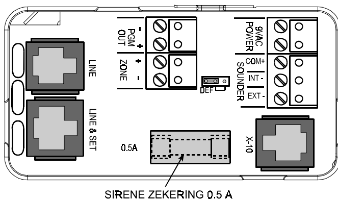
Figuur 32. Locatie van de zekeringen
