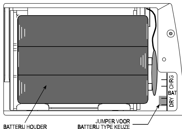
Figuur 31. Jumper in positie voor alkaline batterijen
