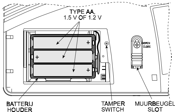
Figuur 5. Batterij houder inclusief batterijen
