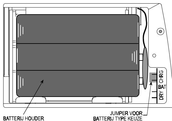
Figuur 4. Batterij type selectie jumper
