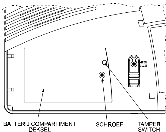
Figuur 3. Batterij ruimte na verwijdering van de deksel.
