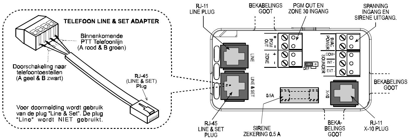
Figuur 9. Overzicht aansluitingen
