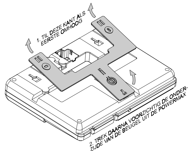
Figuur 7. Losmaken van de beugel
