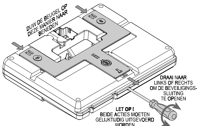
Figuur 6. Het losmaken van de greep
